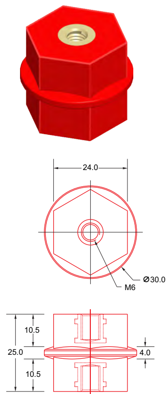
SMV - 0625 (M6) Pkg.: 100; Wt.: 2.200
