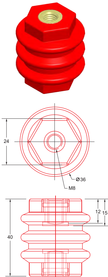
SMV - 0830 (M8) Pkg.: 50; Wt.: 2.500
