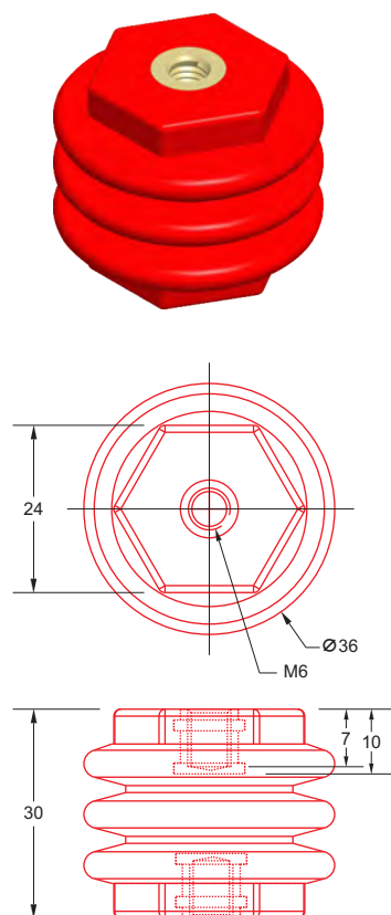
SMV - 0630 (M6) Pkg.: 50; Wt.: 2.250
